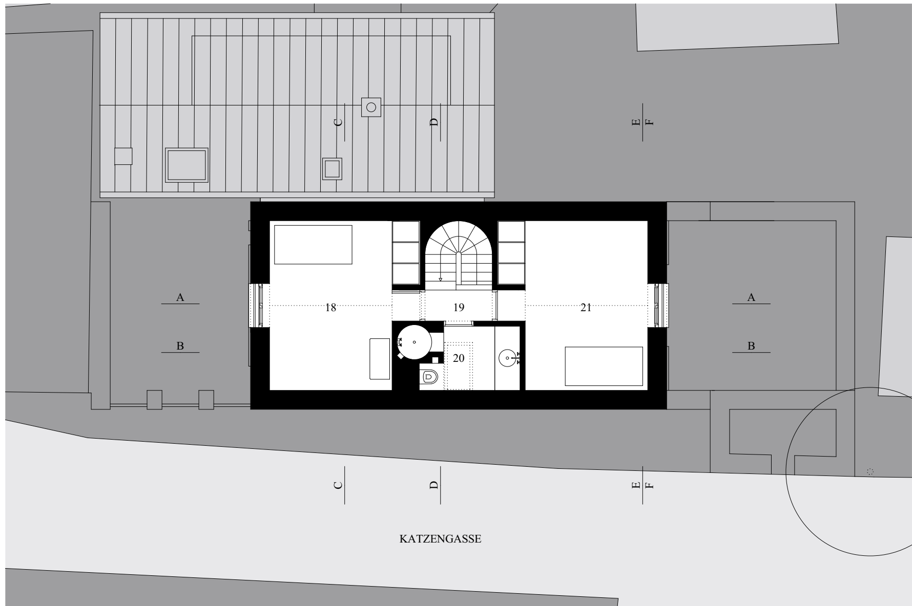
03 GRUNDRISS DG M.1:100 LEGENDE: 18 ZIMMER, 19 FLUR, 20 BAD, 21 ZIMMER
