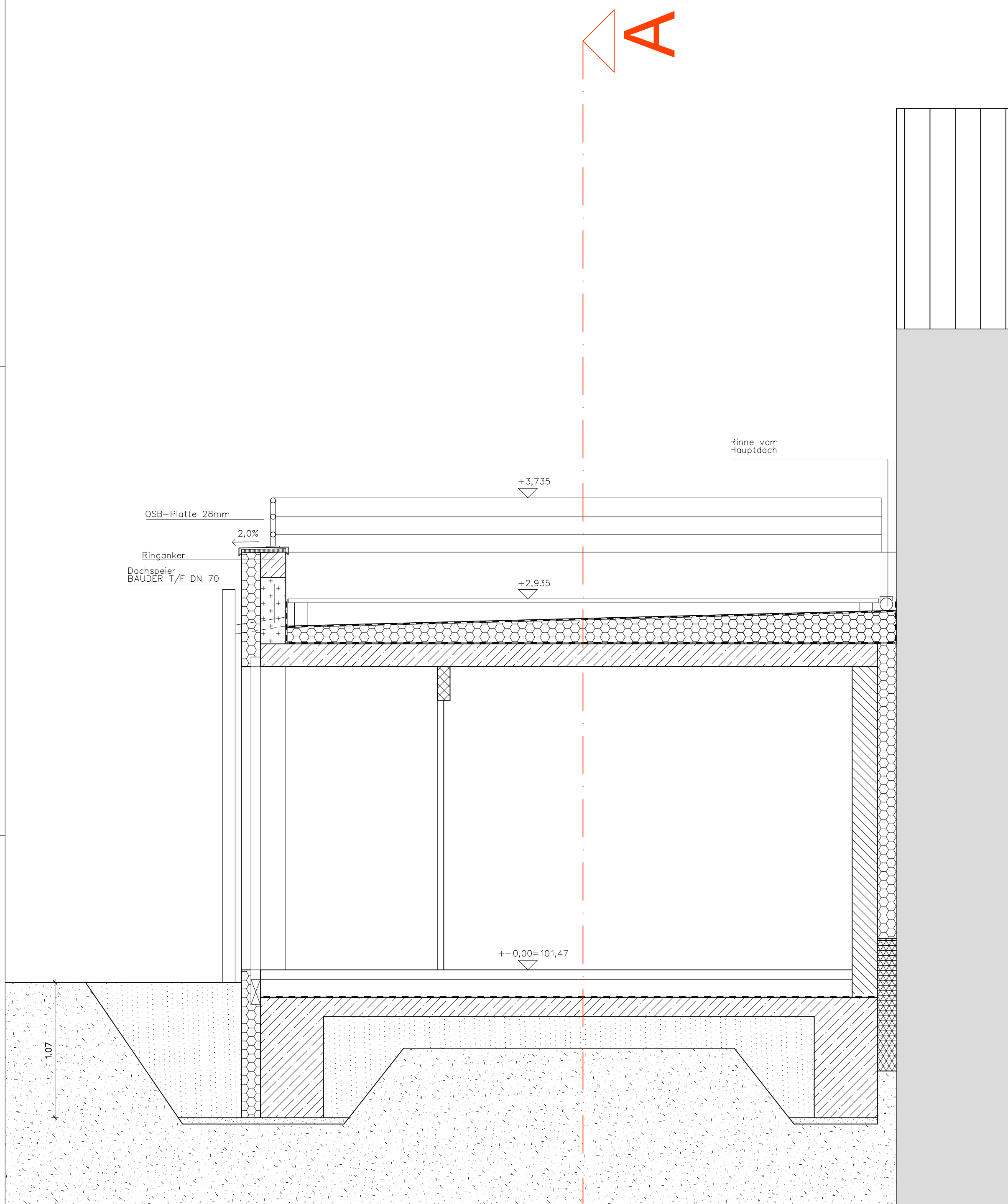
Schnitt DD
