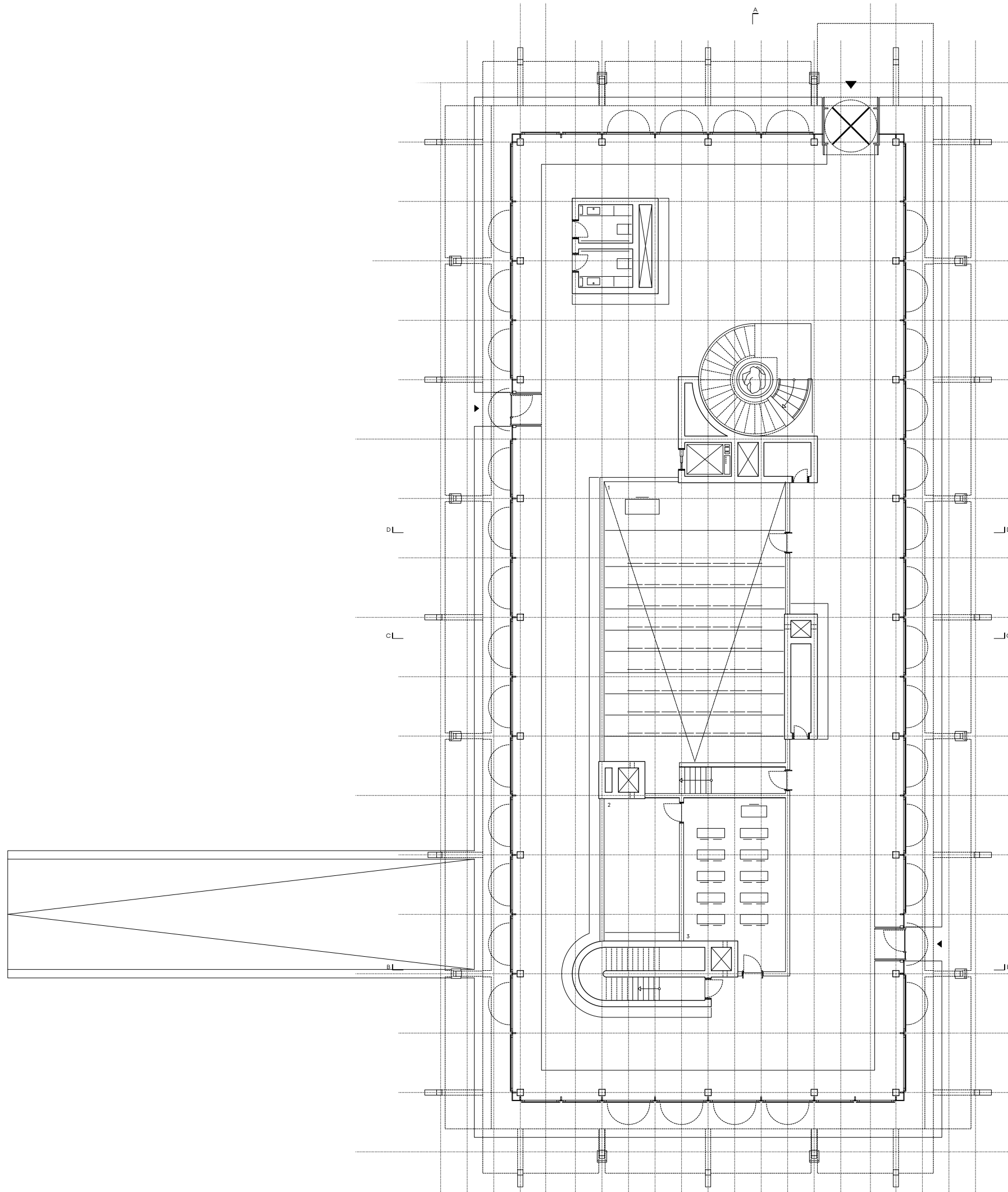
Fakultät Grundriss Erdgeschoss
