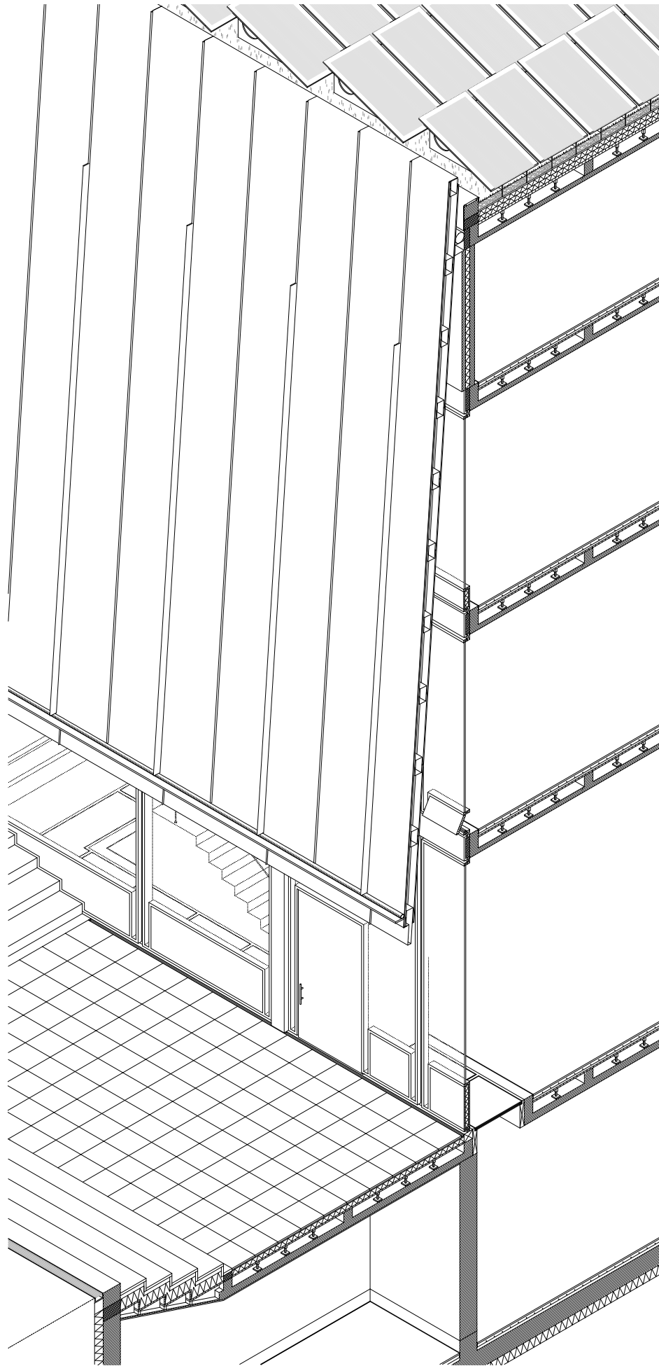
Archiv Fassadendetail
