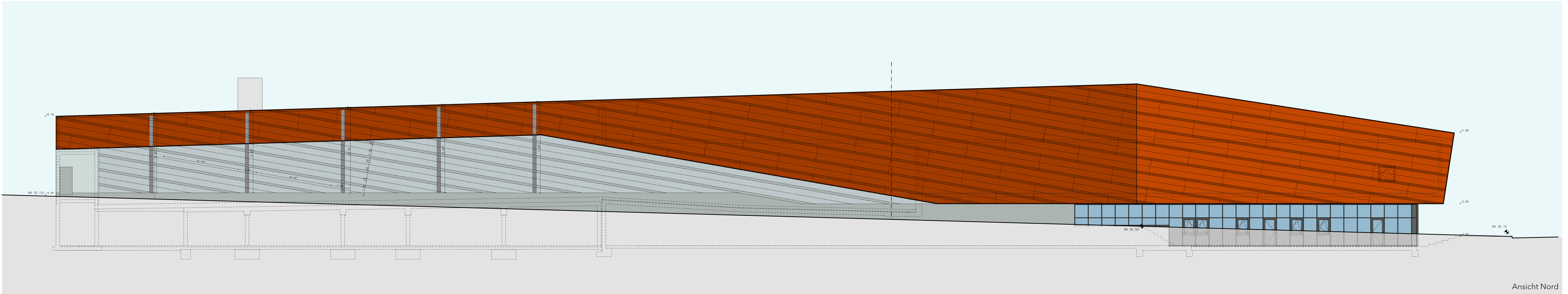
Schnitt 7-7 | Ansicht Nord - M 1_100
