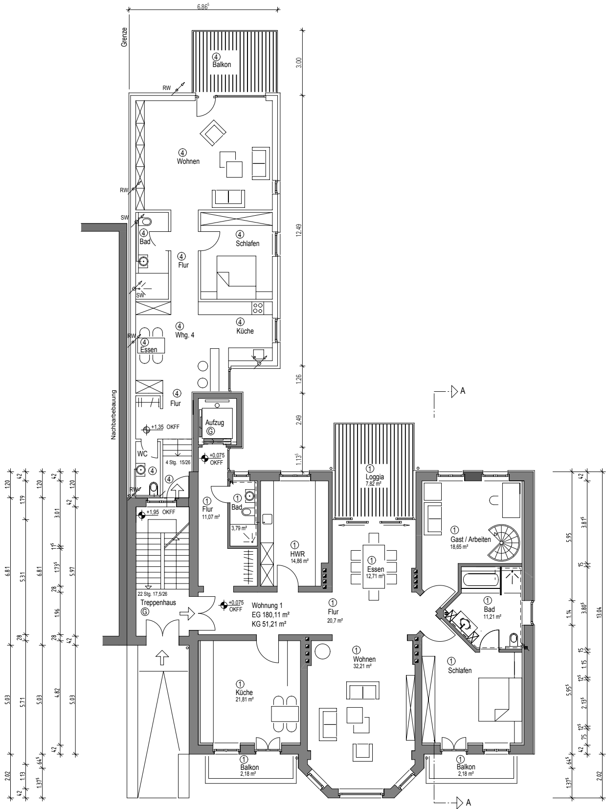
Grundriss Erdgeschoss
