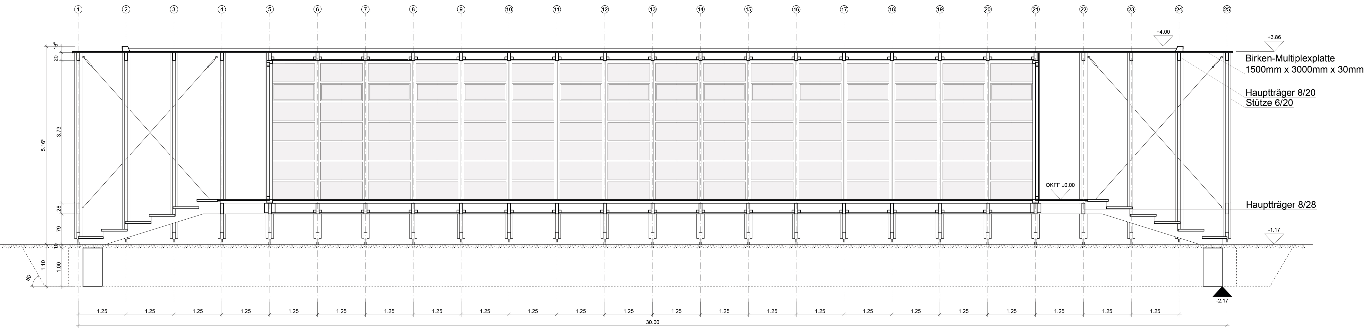
SCHNITT 1:50
