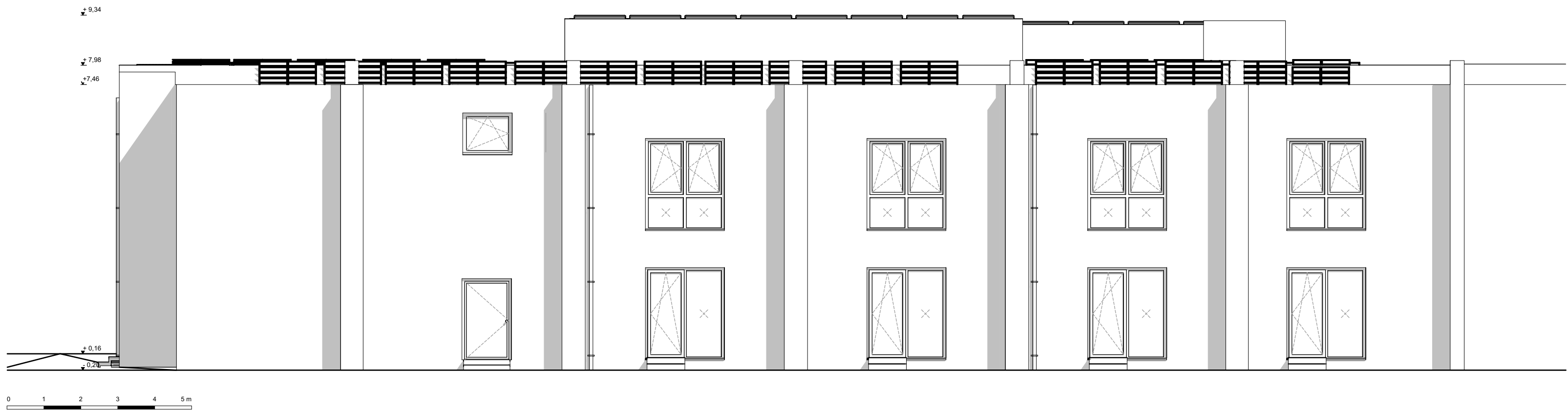
Ansicht Süd
