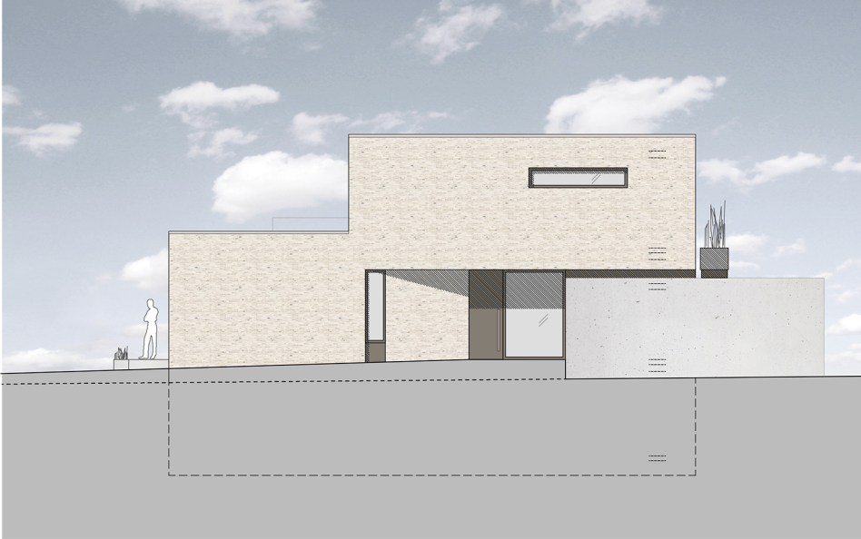
ANSICHT OST
