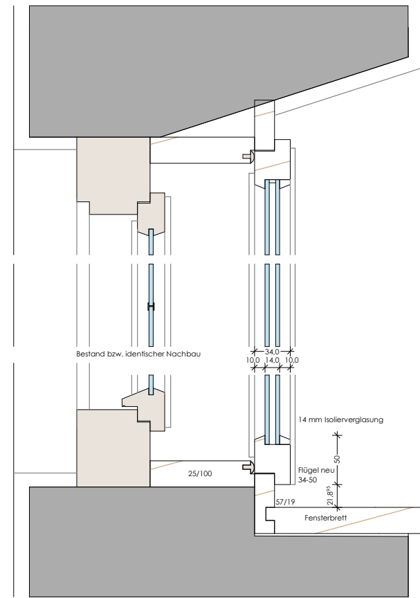
Längsschnitt M 1 | 5
