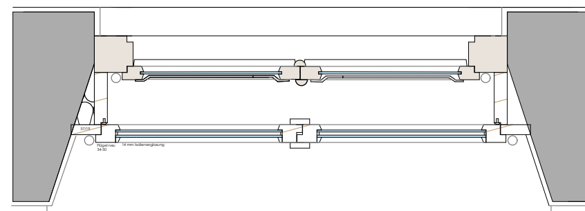
Ansichten Grundriss Schnitt M 1 | 10
