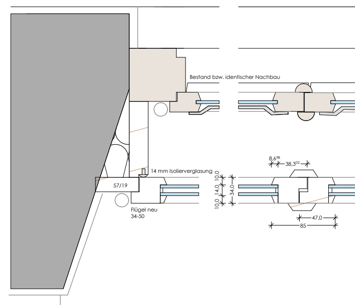
Querschnitt M 1 | 5
