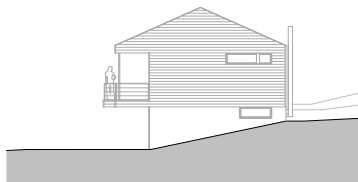
ANSICHT OSTEN
