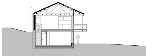
QUERSCHNITT
