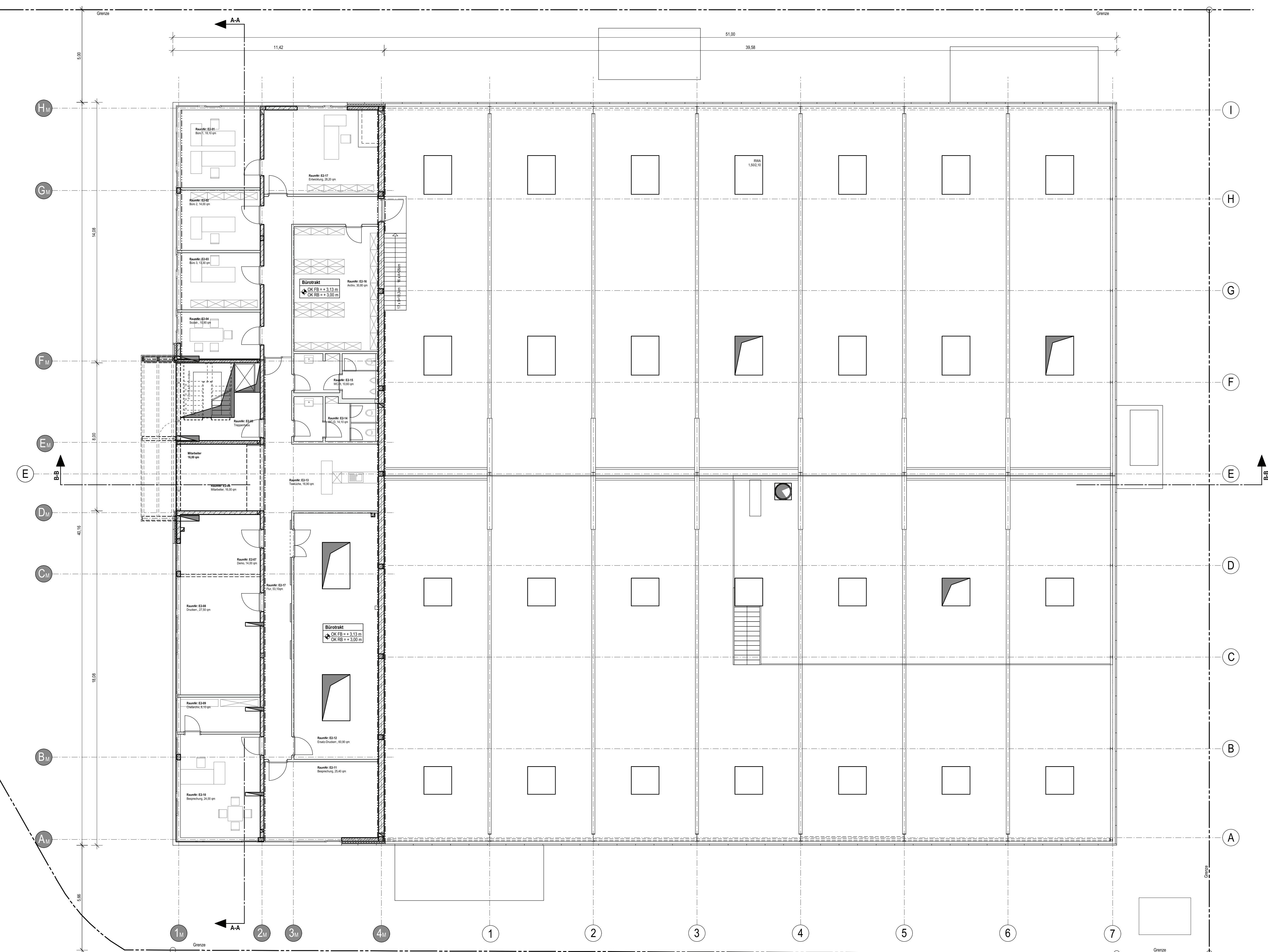
1. Obergeschoss
