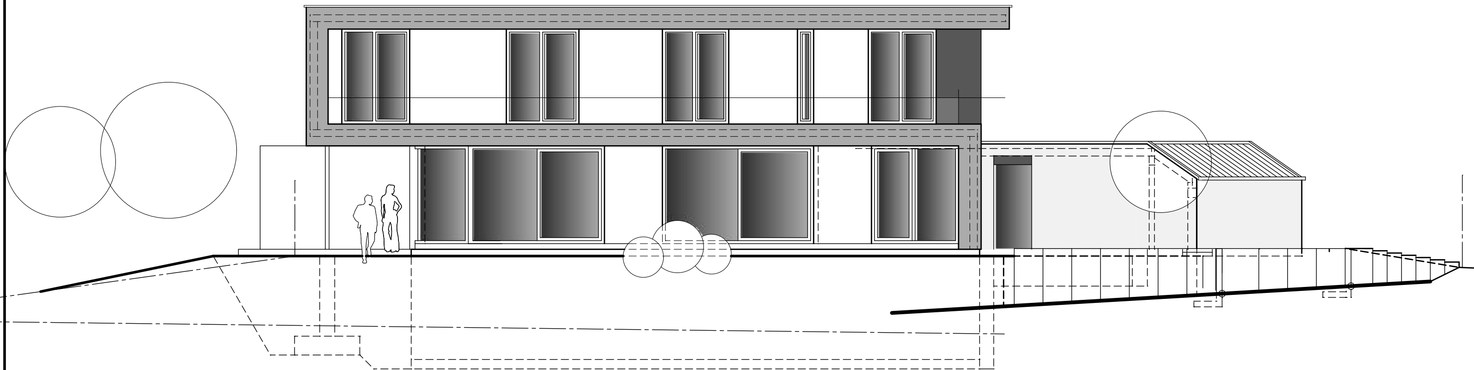
ANSICHT SÜD-OST
