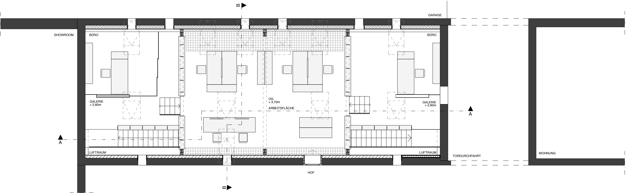
GRUNDRISS OBERGESCHOSS / GALERIE 1:100
