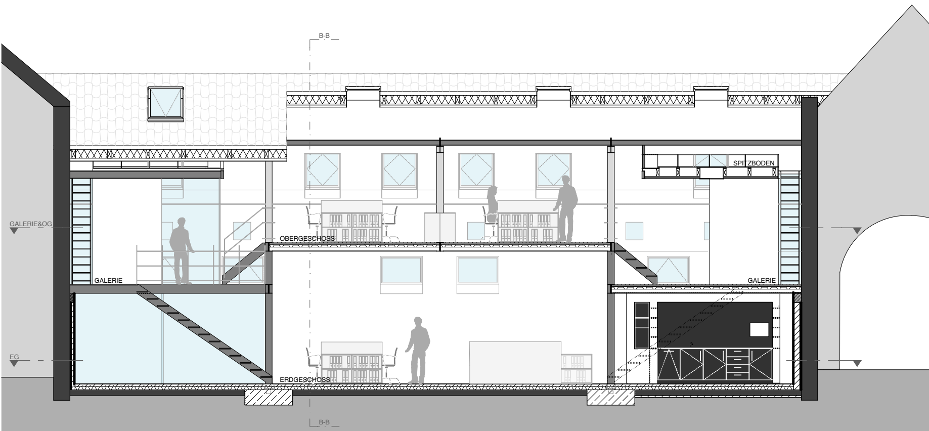
SCHNITT A-A 1:100
