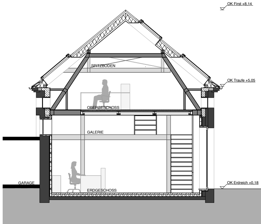
SCHNITT B-B
