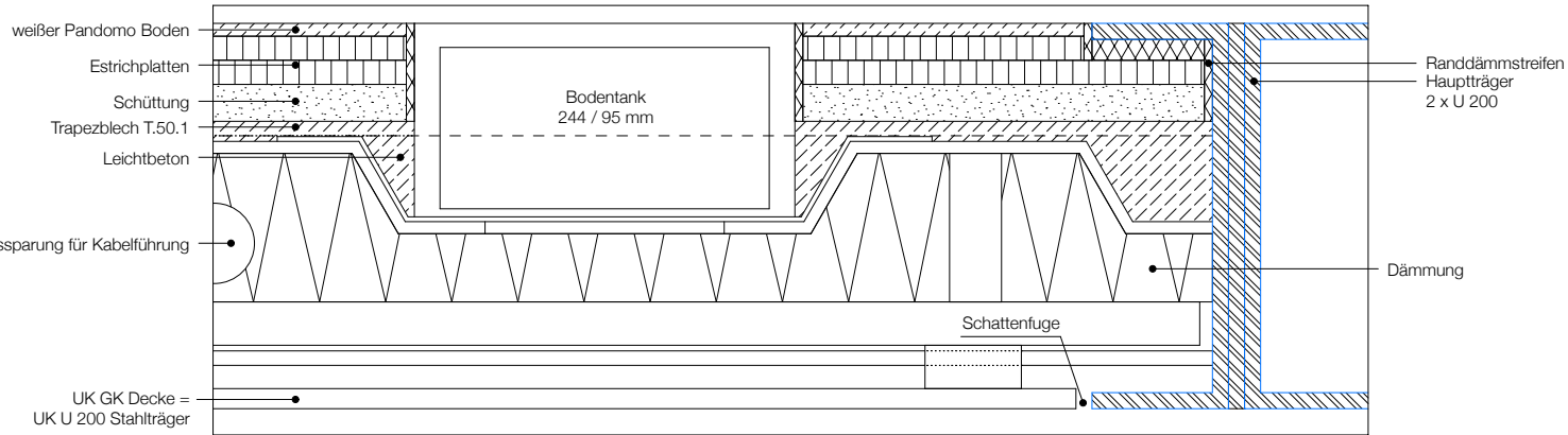
SCHNITT HAUPTTRÄGER 1:5
