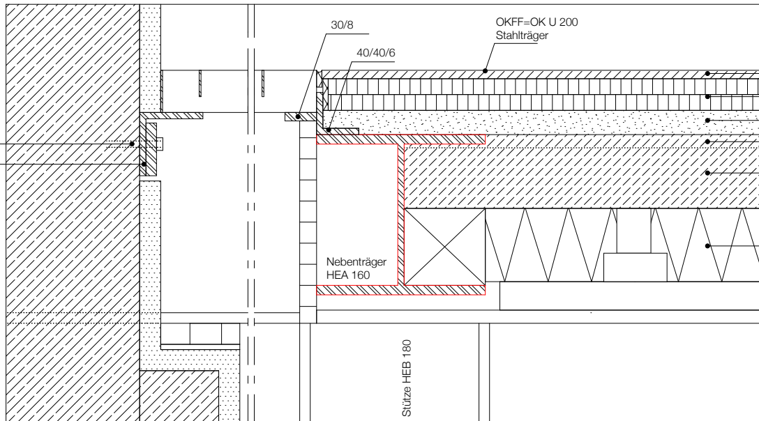
SCHNITT NEBENTRÄGER MIT ANSCHLUSS GITTERROST 1:5
