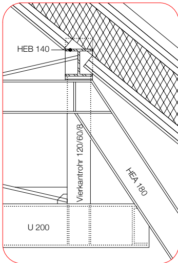
DETAIL SPITZBODEN HÄNGENDE KONSTRUKTION 1:20
