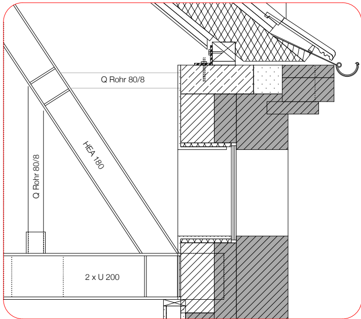
DETAIL WANDANSCHLUSS STAHLRAHMEN 1:20
