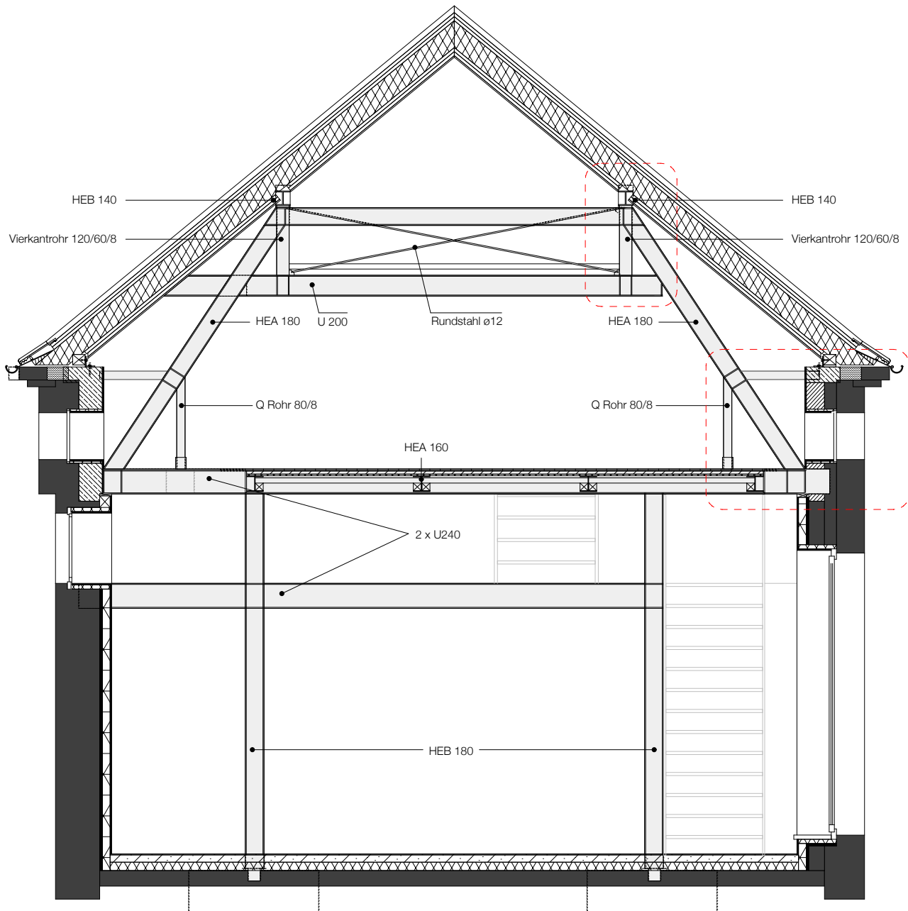
SCHNITT STAHLKONSTRUKTION 1:50
