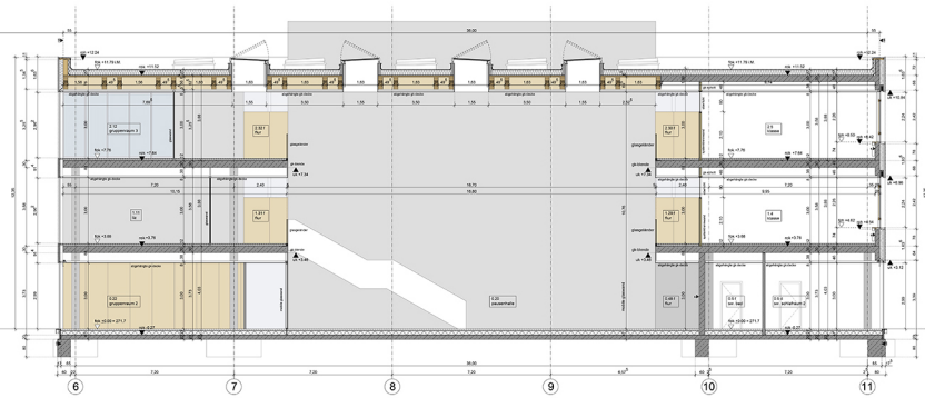
SNITT 1-1
