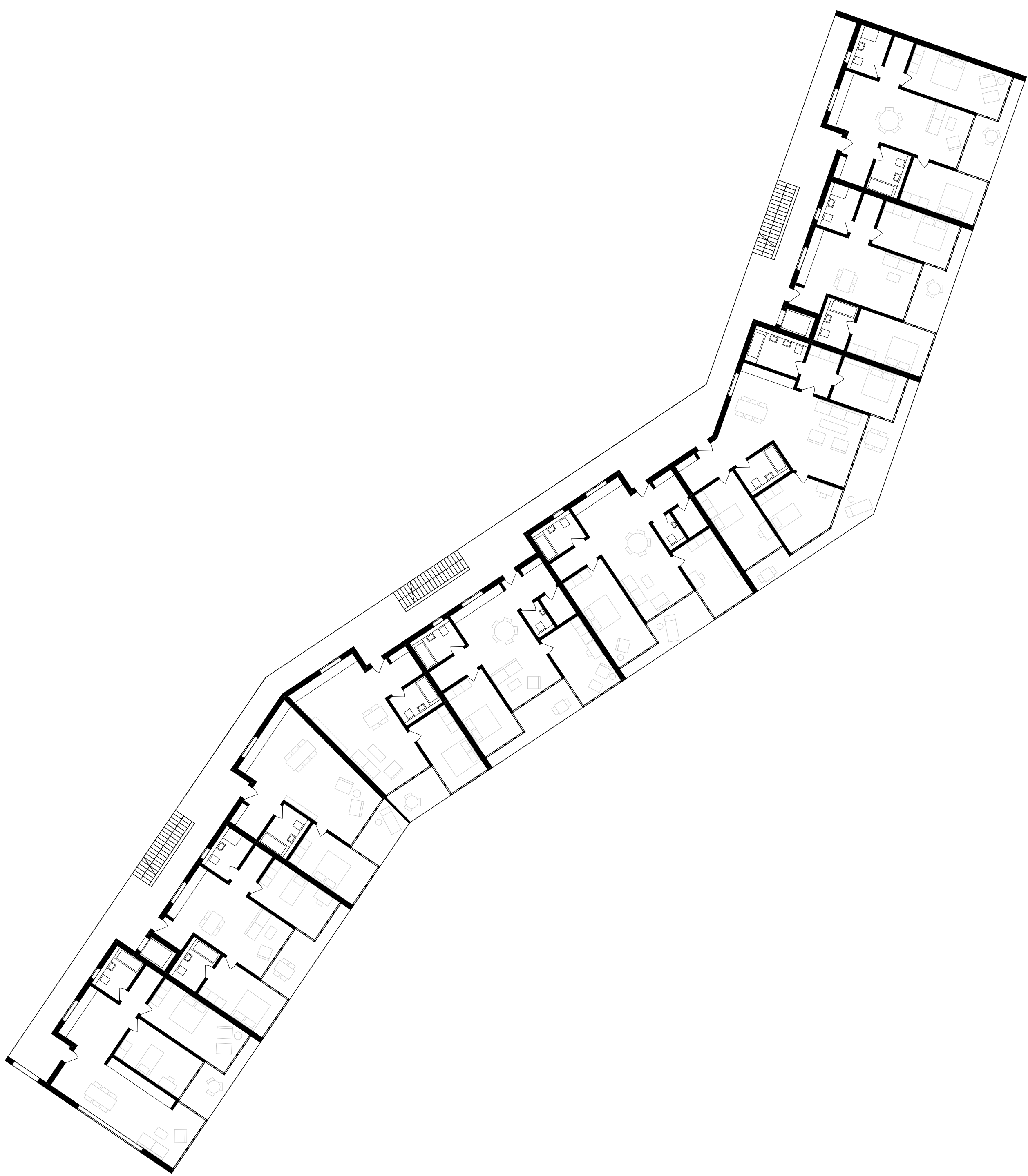
Regelgeschossgrundriss I M 1:200
