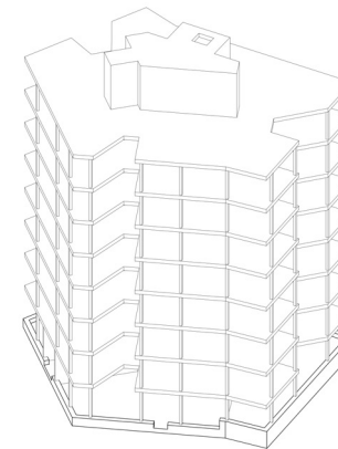
Isometrie Turm Kernstruktur
