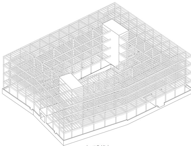
Isometrie Block Nord Kernstruktur
