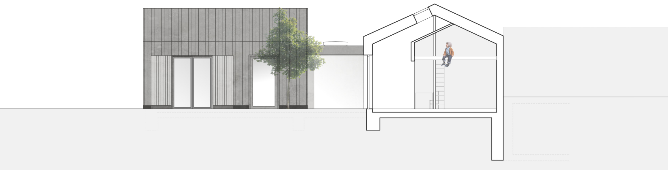
schnitt a-a | m 1:100
