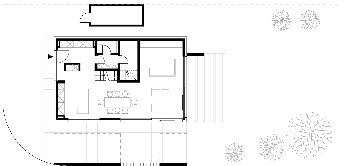
GRUNDRISS EG
