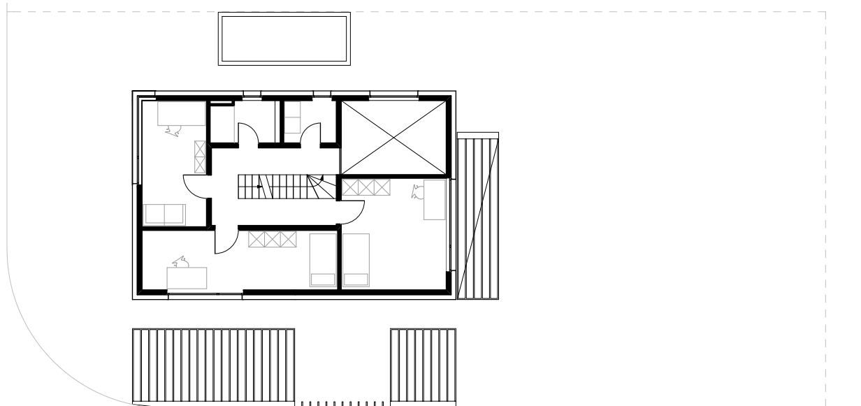
GRUNDRISS OG
