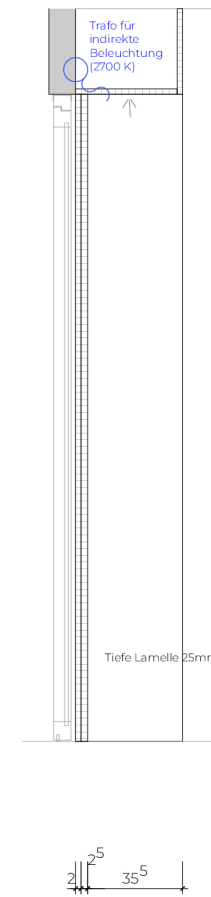
Schnitt C-C
