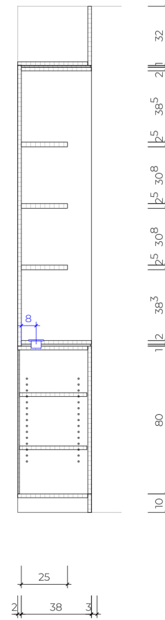
Schnitt B-B
