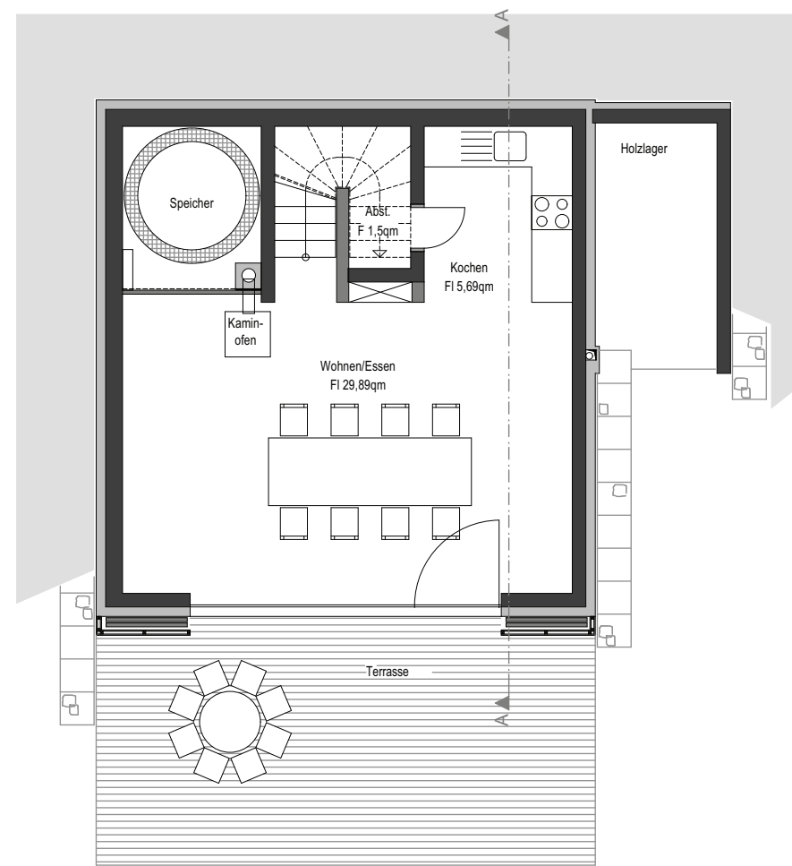
Grundriss Erdgeschoss 1:100
