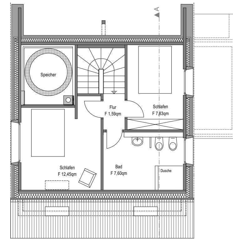
Grundriss Dachgeschoss 1:100
