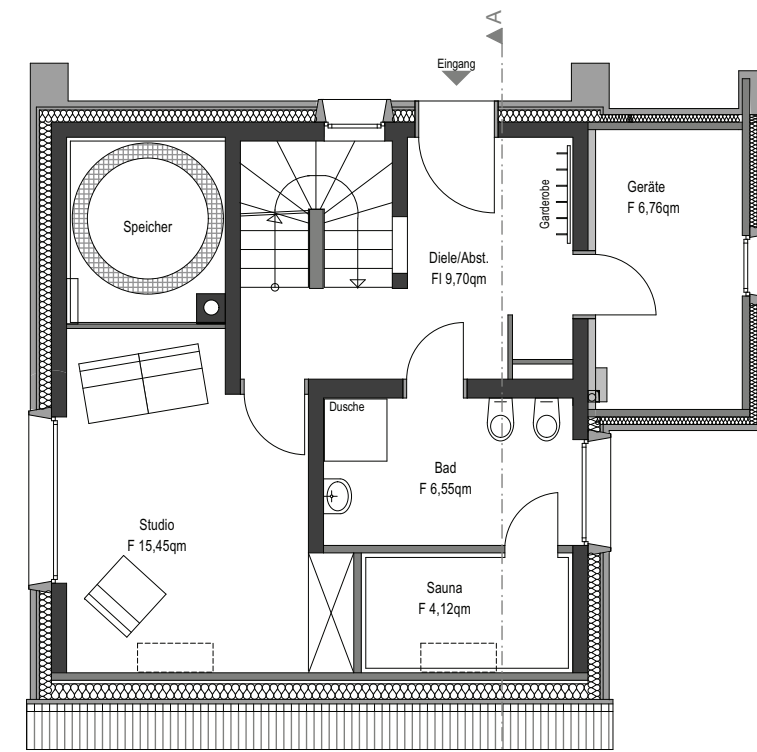
Grundriss 1. Obergeschoss 1:100
