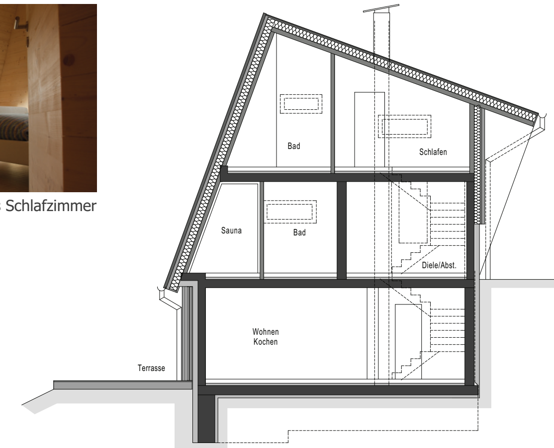
Schnitt 1:100
