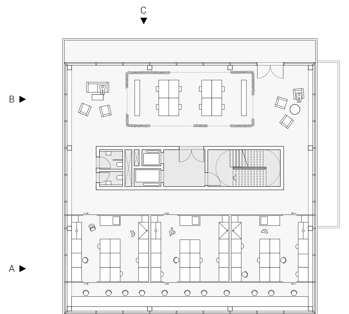
6.0G Labore und Aufenthaltsbereiche
