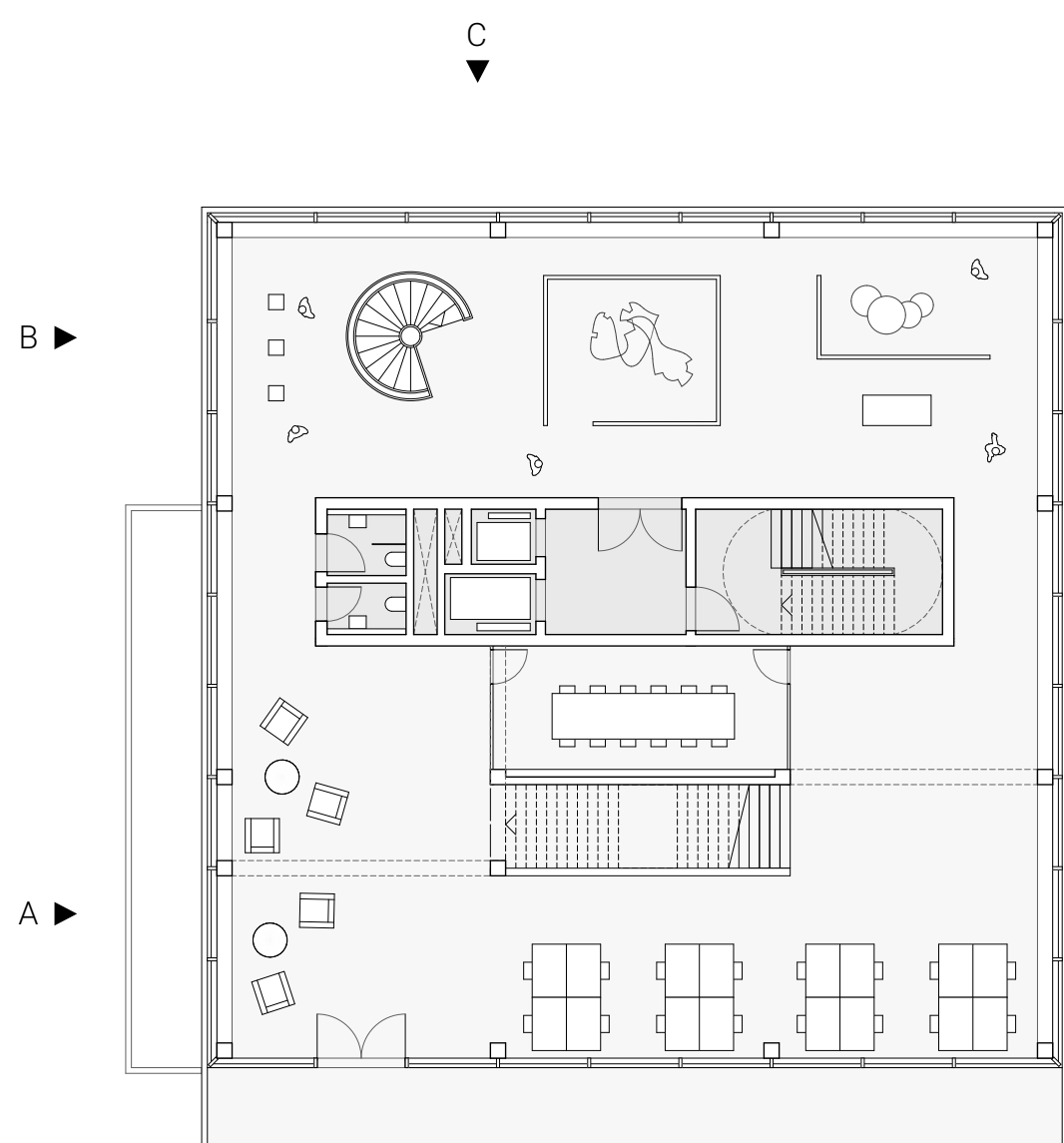
4.0G Leseräume und Ausstellungsfläche
