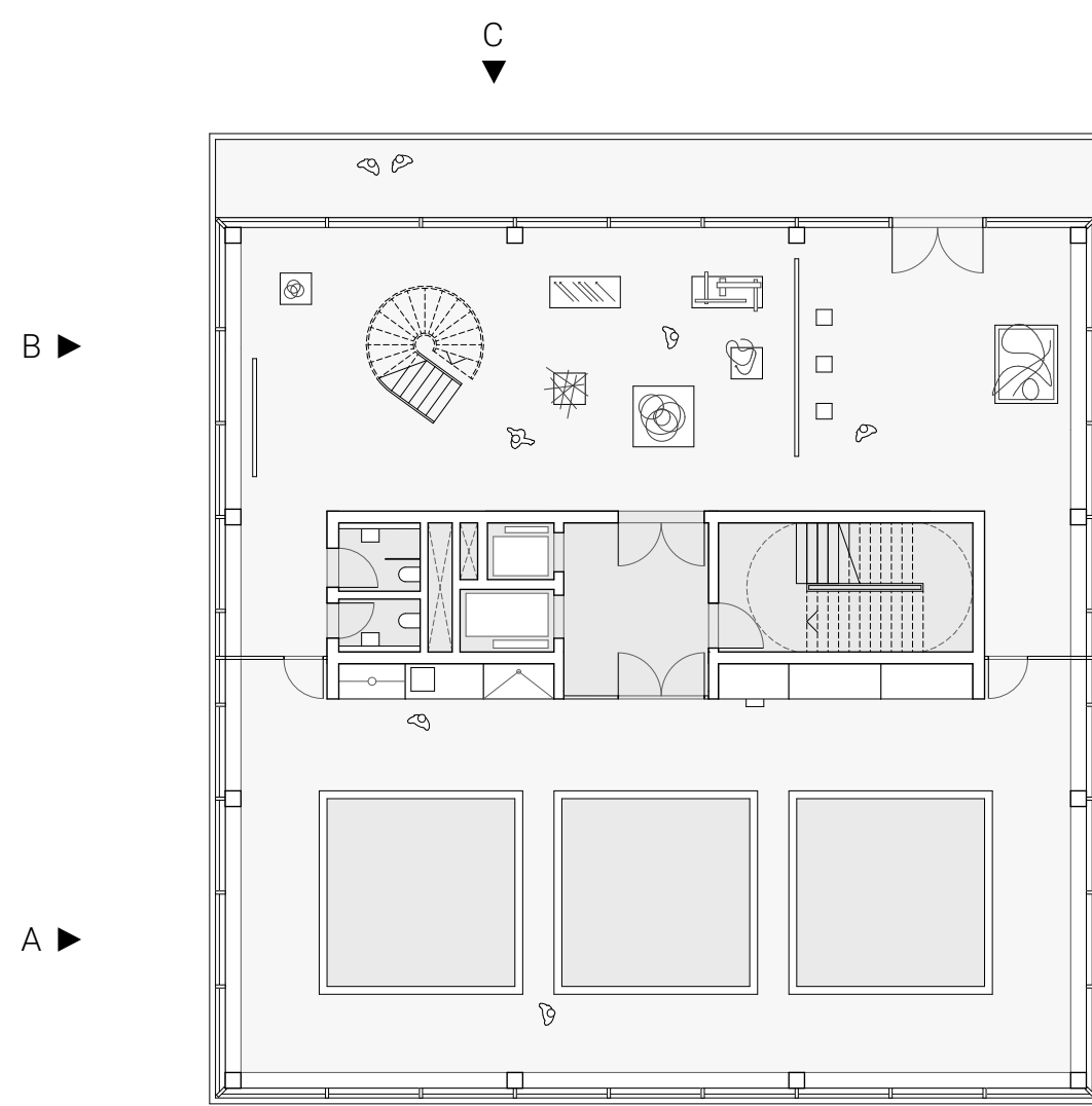
2.0G Wasserbecken und Ausstellungsfläche
