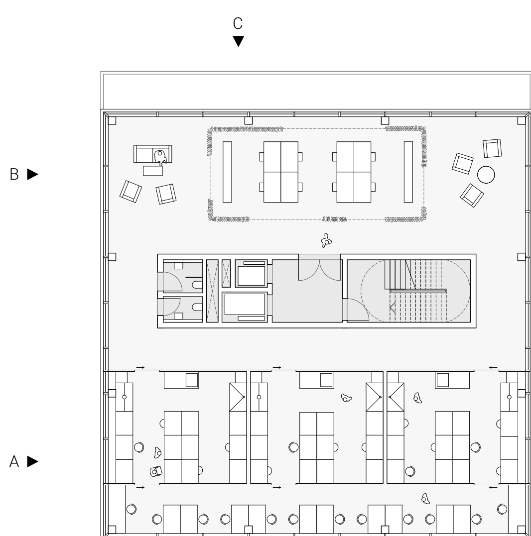
7.0G Labore und Aufenthaltsbereiche
