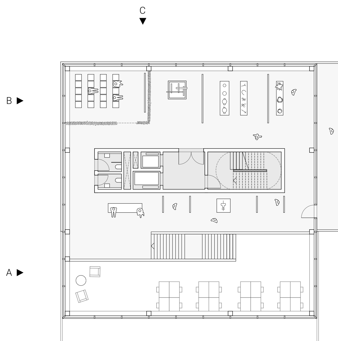
5.0G Luftraum und Ausstellungsfläche mit Kino
