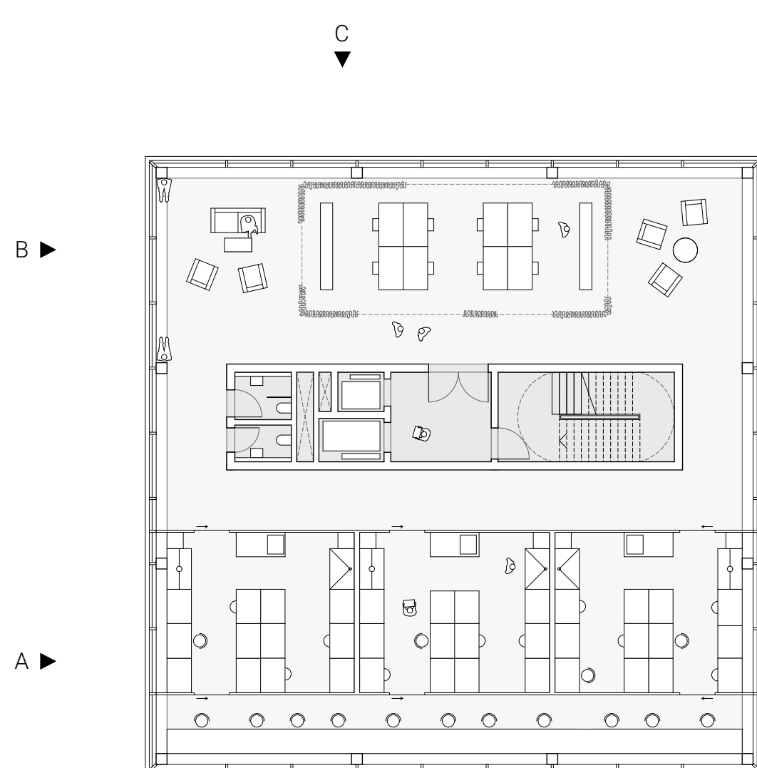
8.0G Labore und Aufenthaltsbereiche
