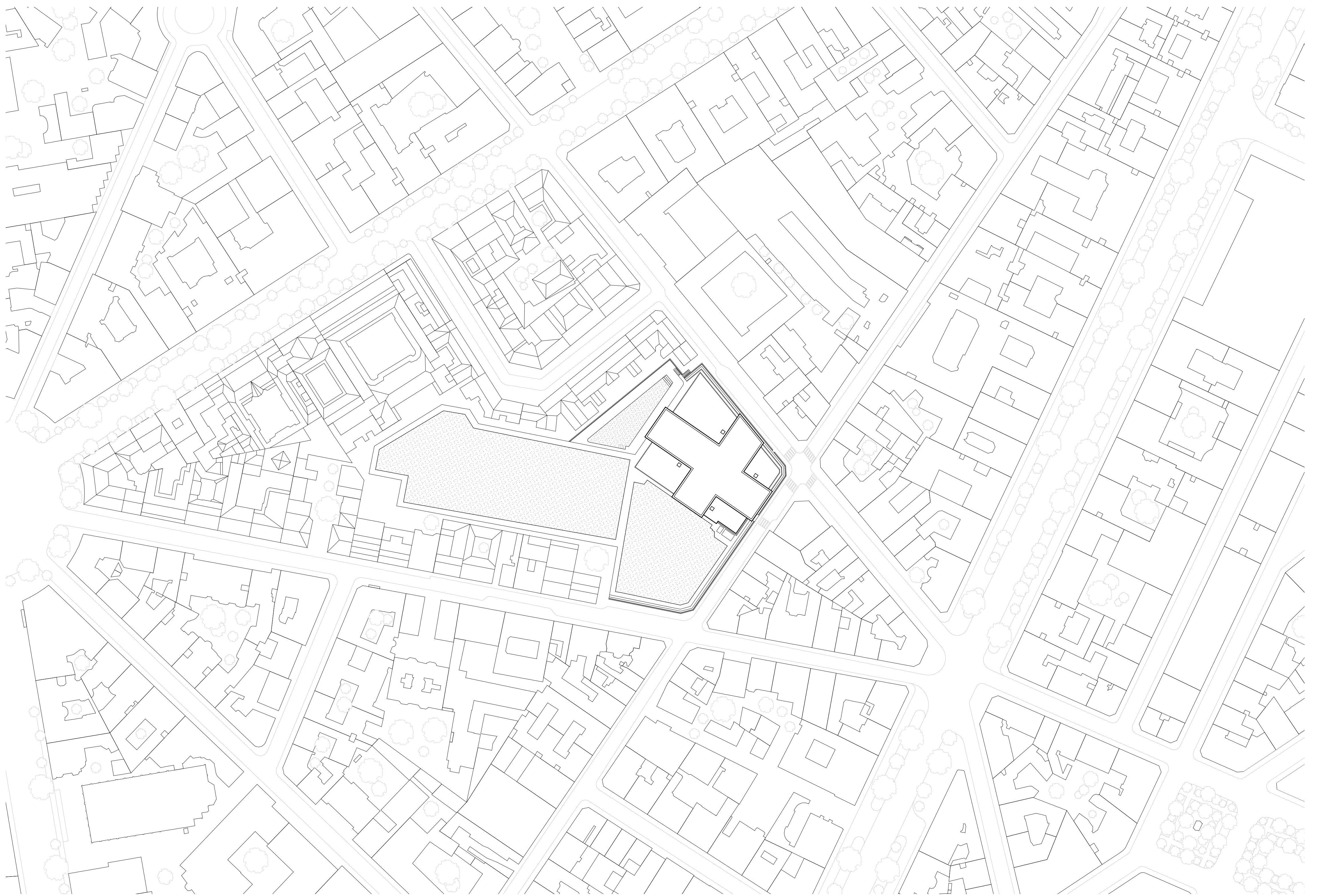
Lageplan 1_1000
