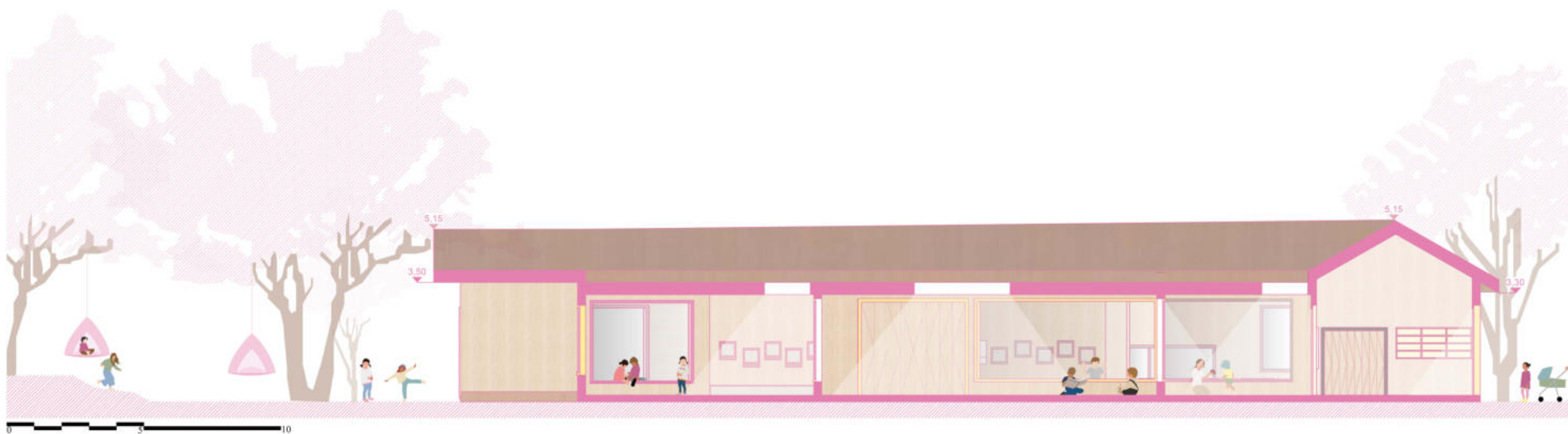
SCHNITT A-A
