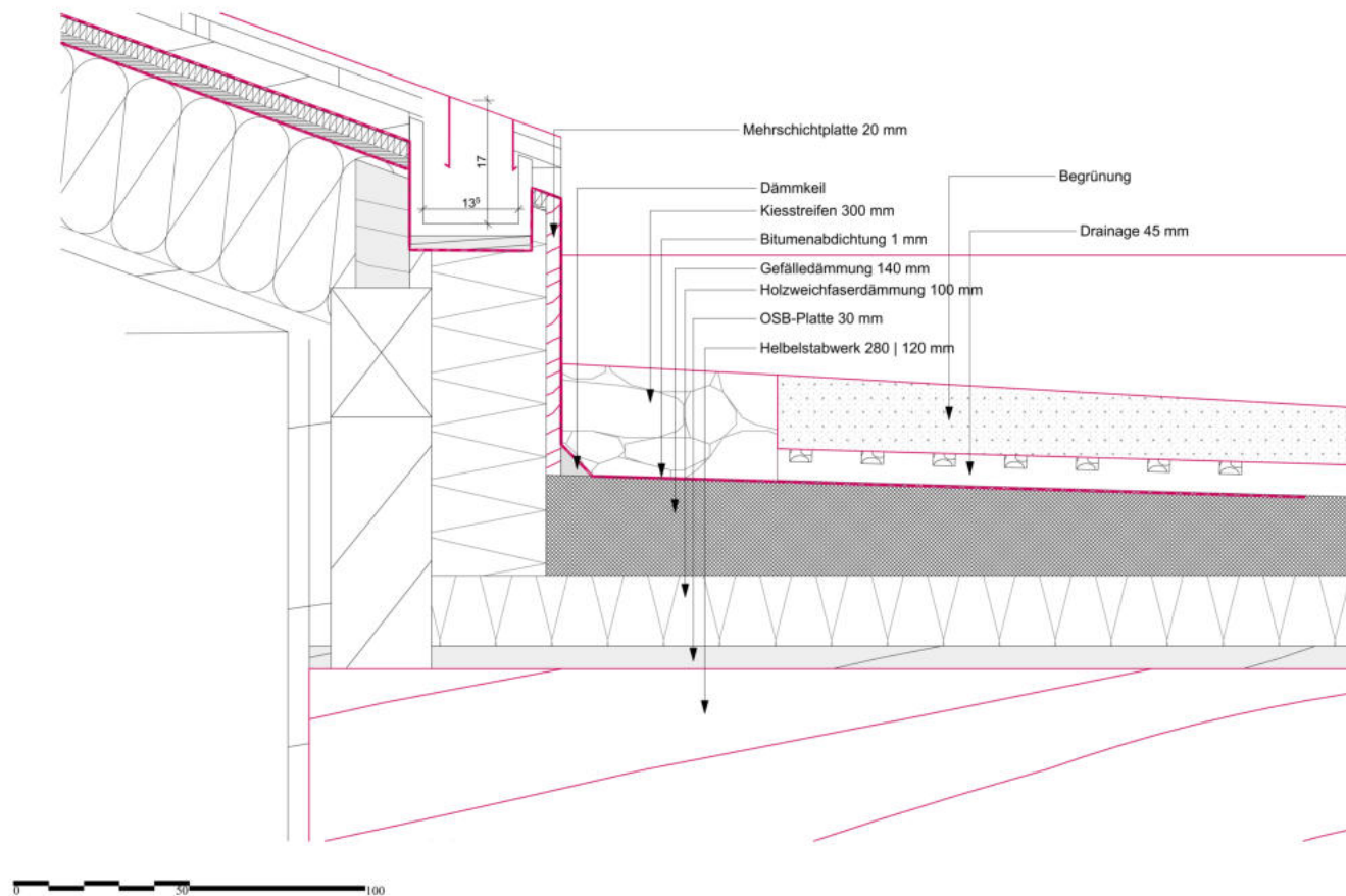
DACHDETAIL KONSTRUKTION
