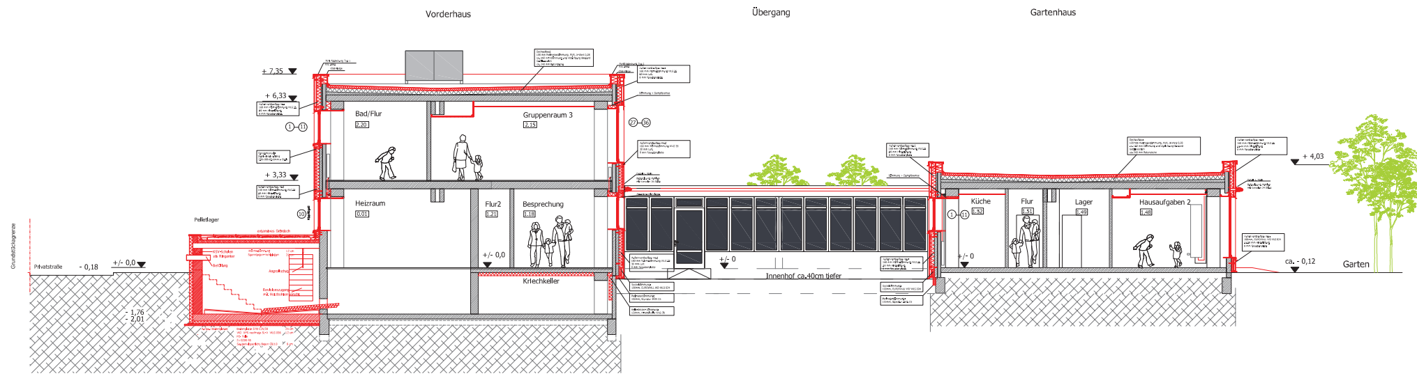
Schnitt B-B
