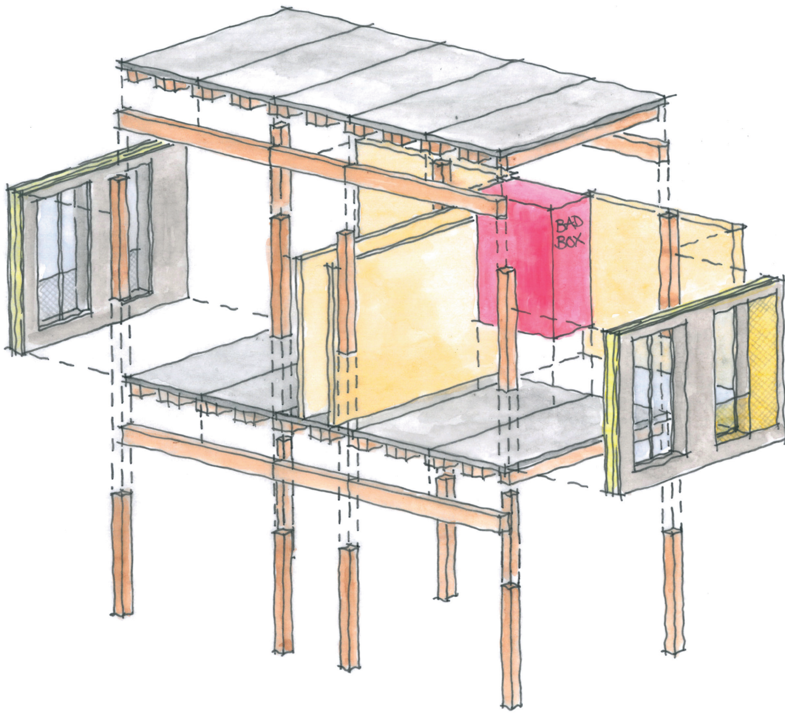
KONZEPT I AUF- UND ABBAUPRINZIP
