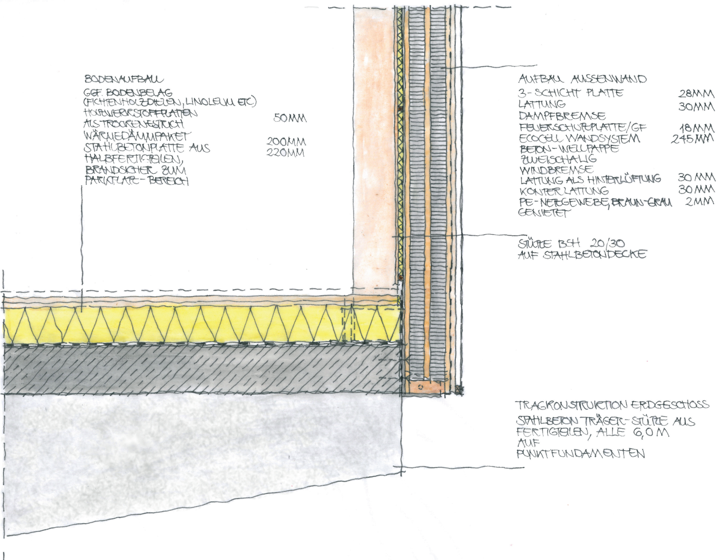
DETAIL I FASSADENSCHNITT I M 1/20
