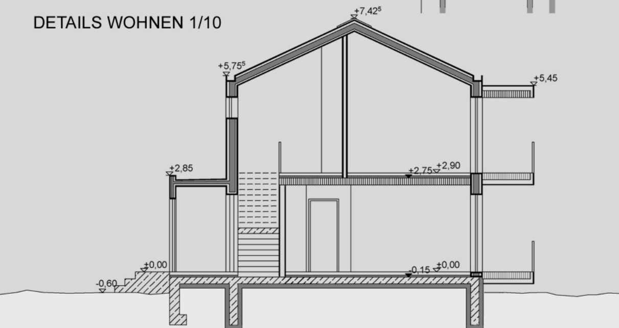
SCHNITT 1/100
