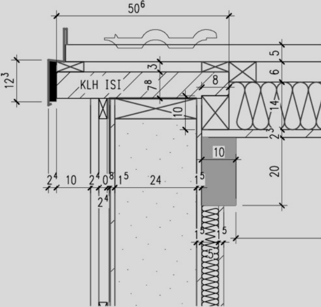
DETAILS WOHNEN 1/10
