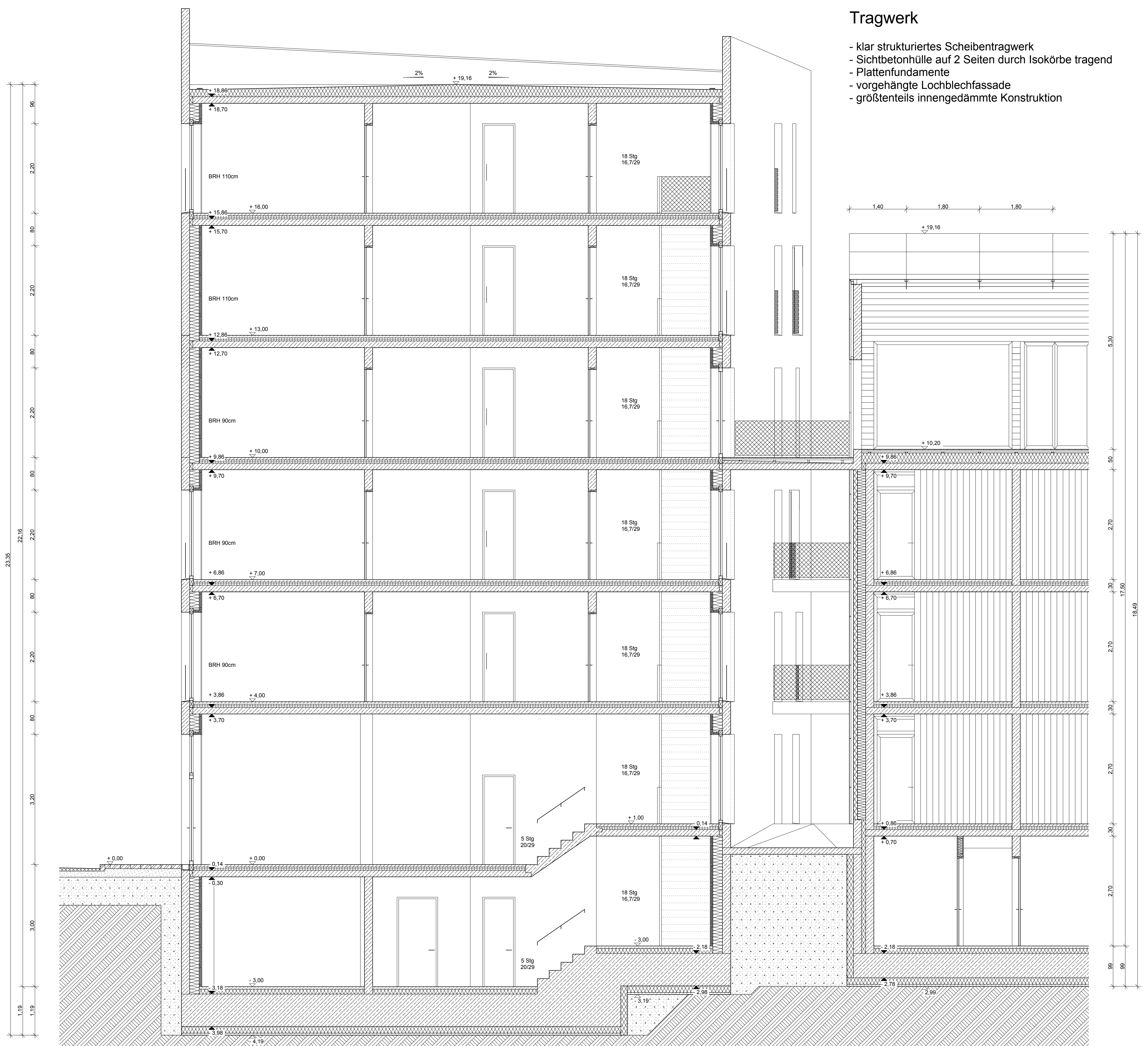
Teilschnitt A
