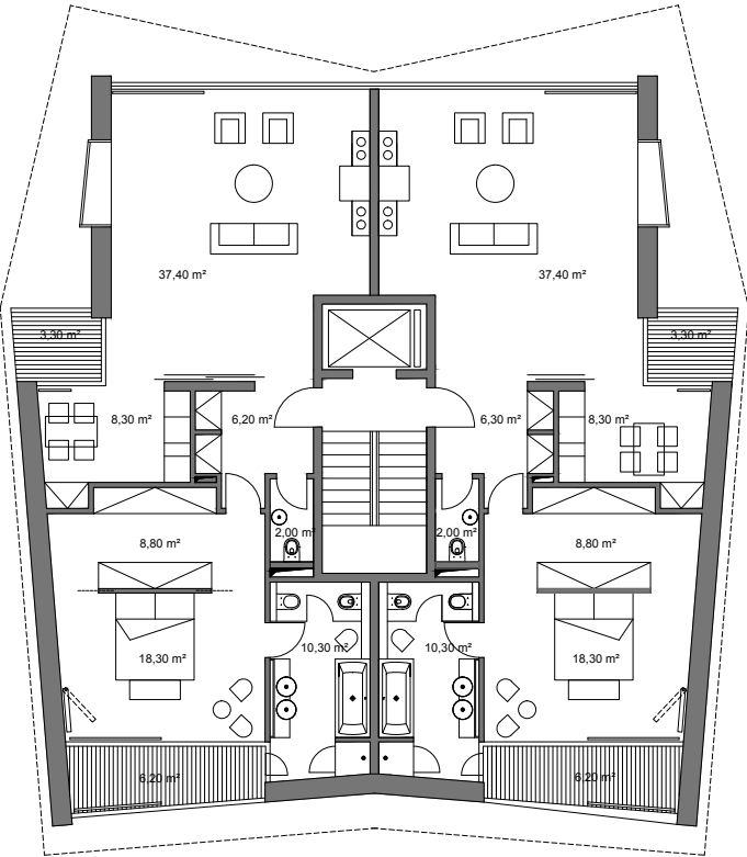
2 - ZIMMERWOHNUNGEN 100 m²
