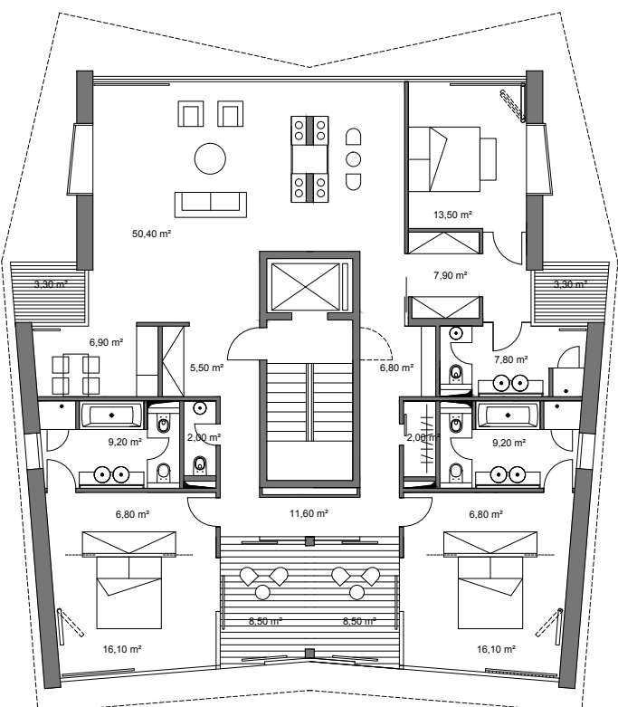
4 - ZIMMERWOHNUNG 200 m²
