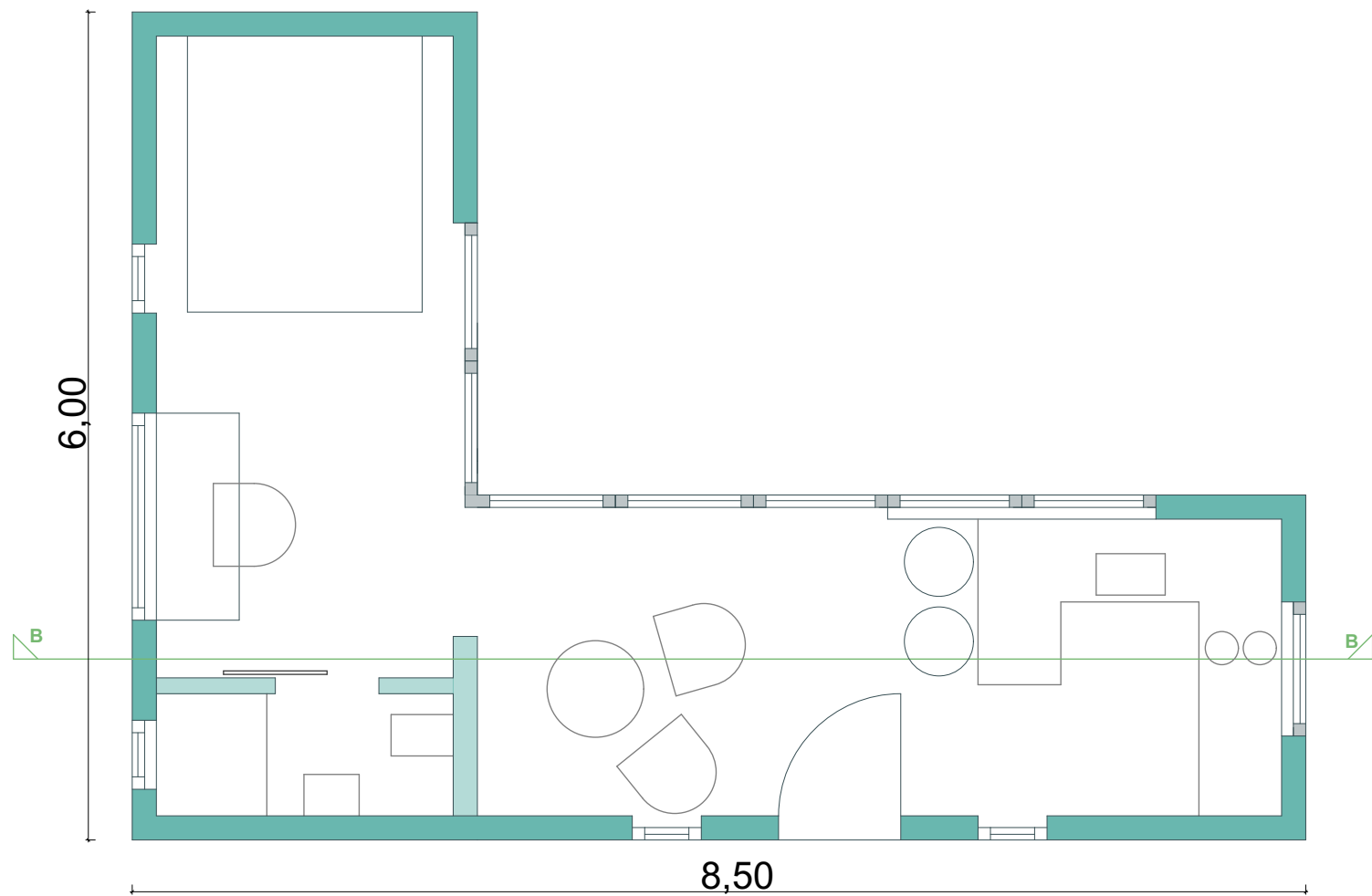
Grundriss EG 2
