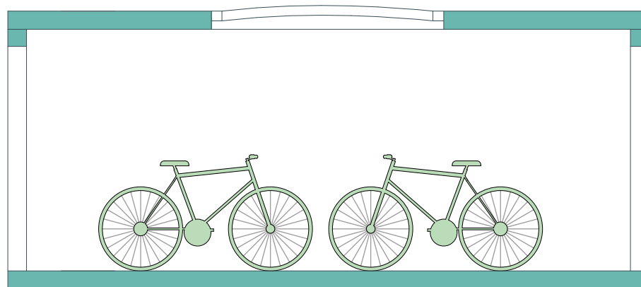
Schnitt D-D Garage
