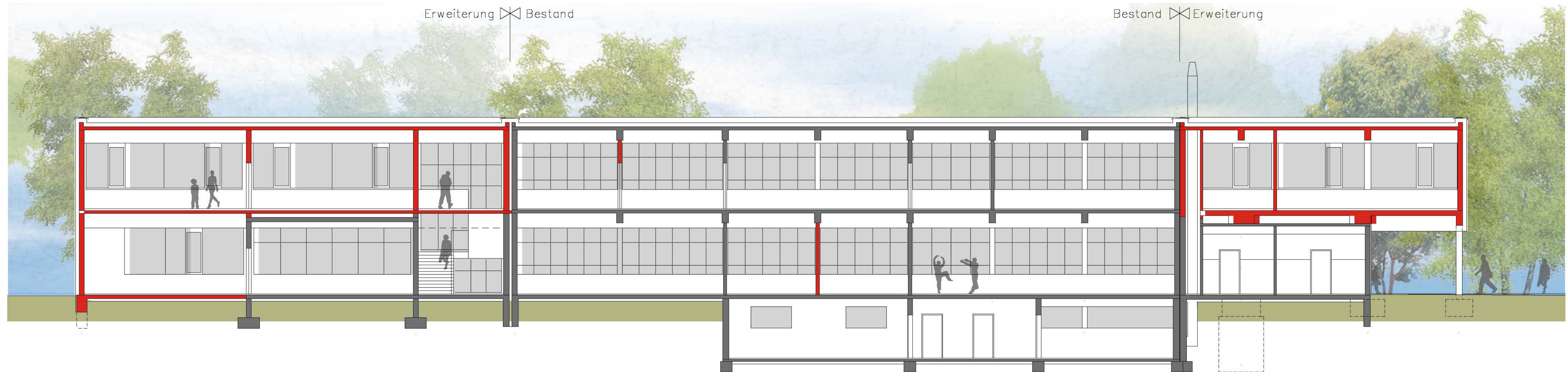
LANGSSCHNITT B-B'
