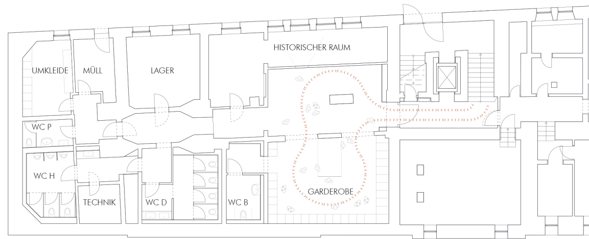
GRUNDRISS UG
