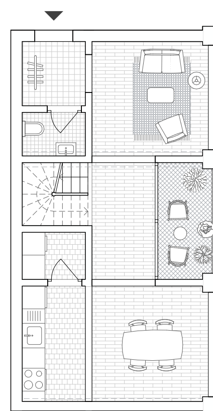
WT6 Duplex 3 Zimmer 85 qm
