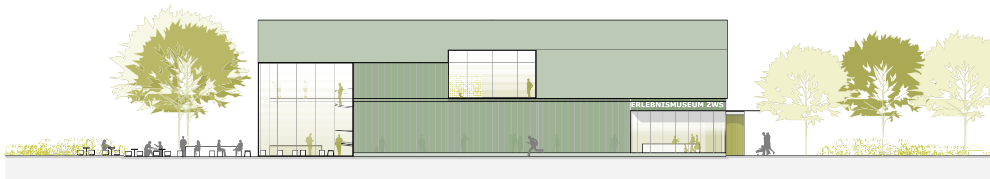
Ansicht Ost
