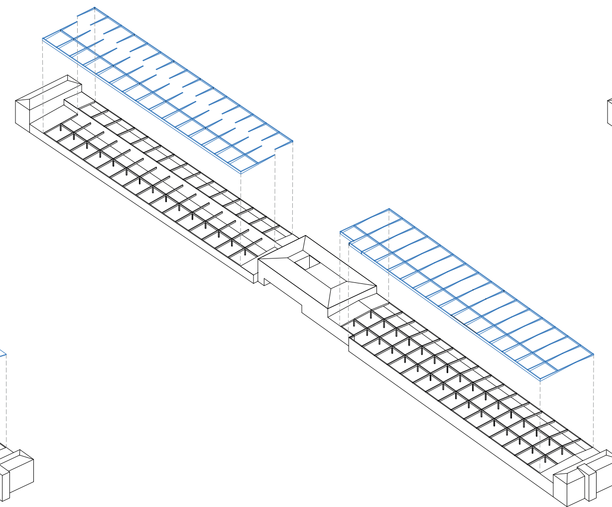
03 AUSGLEICH DACHNEIGUNGEN
