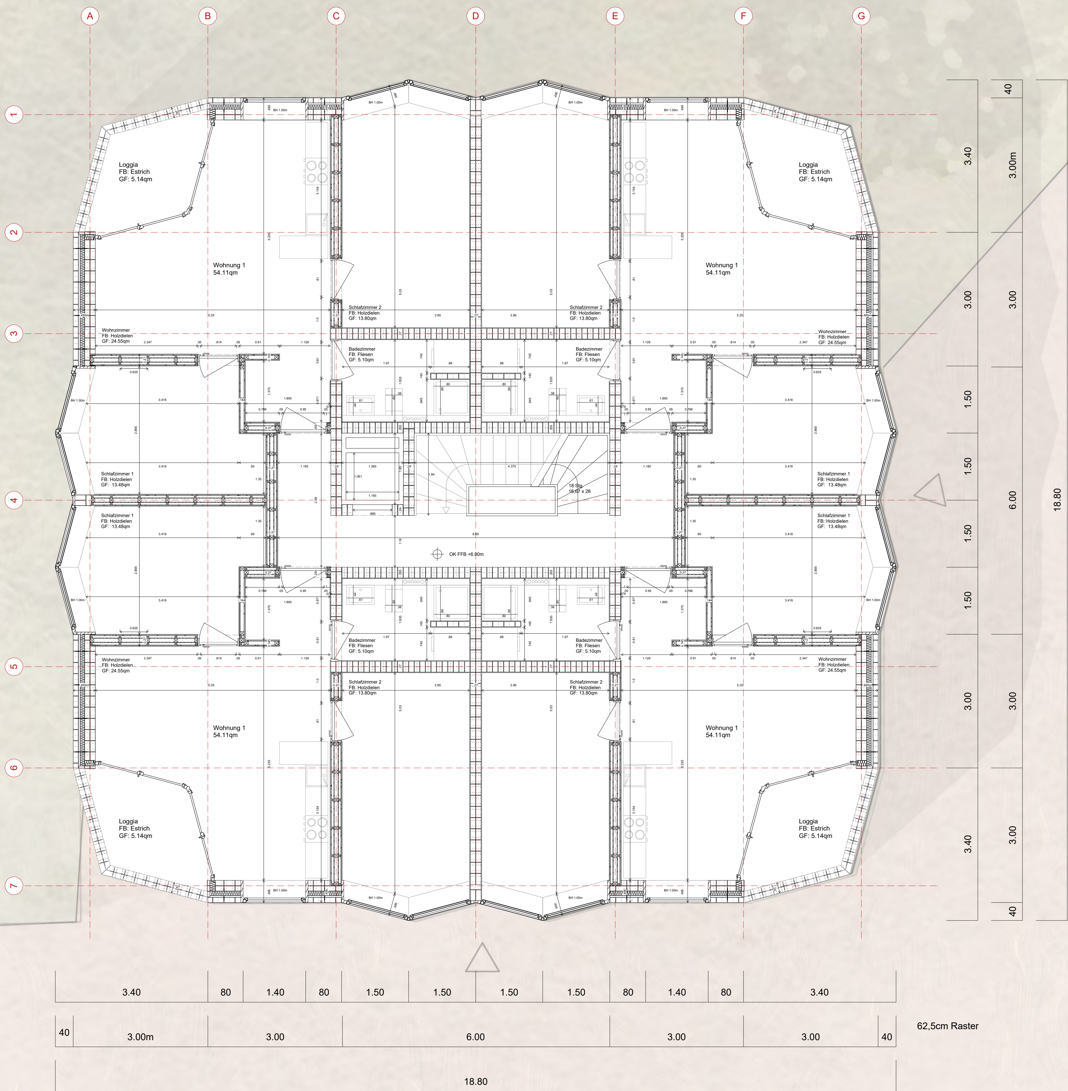
Werkplan 1:50 Wohnungsregelgeschoss
