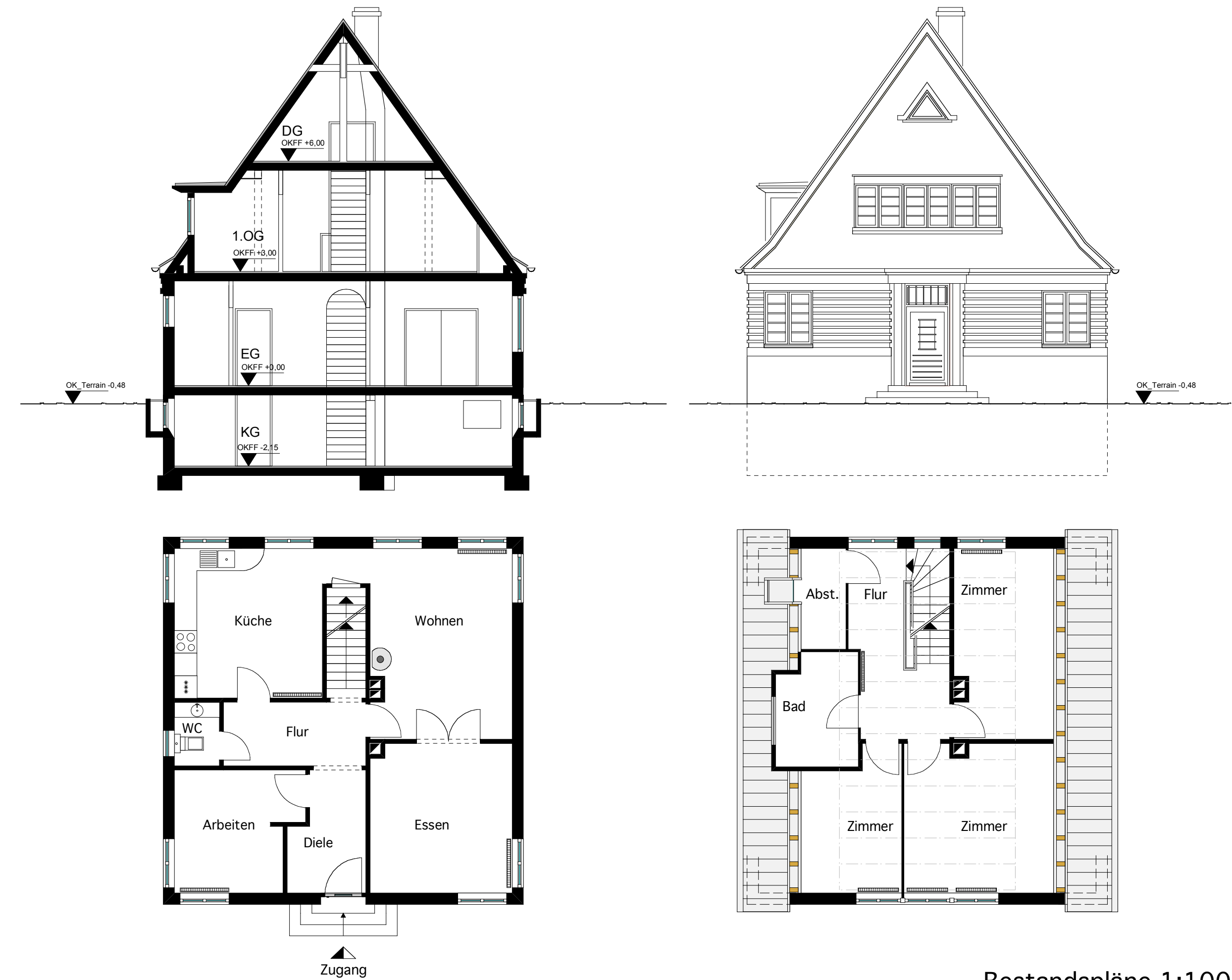
Bestandspläne 1:100
