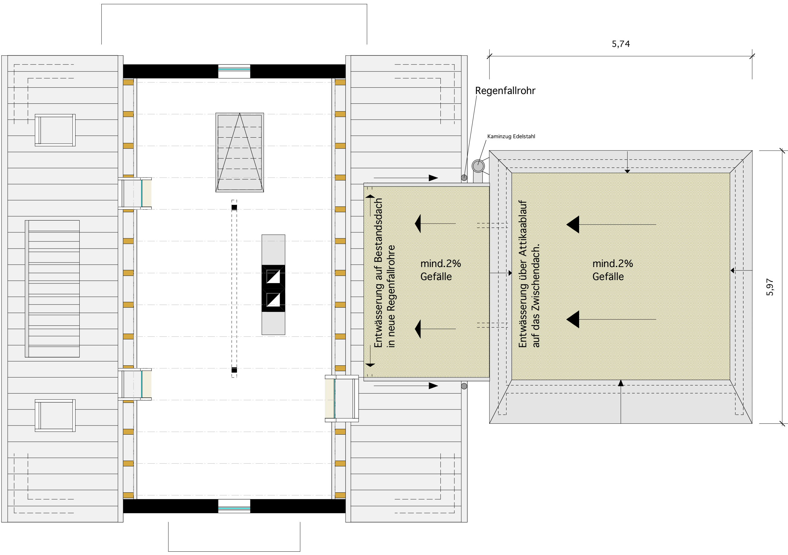
Grundriss Dachaufsicht
