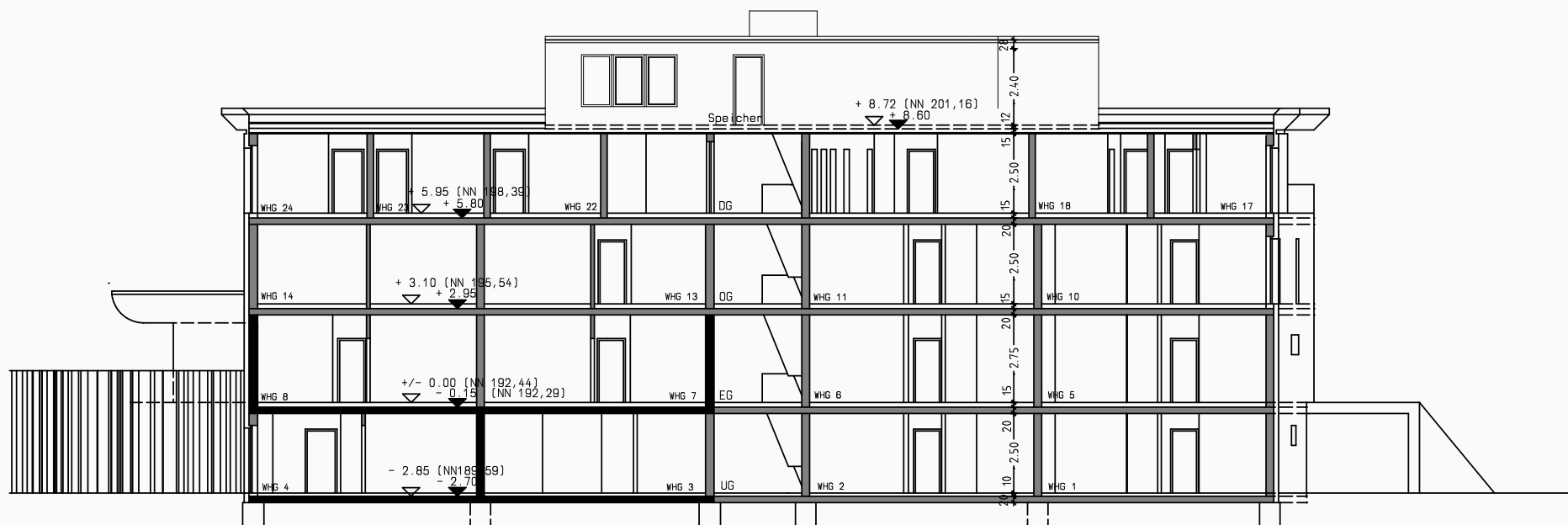
Schnitt
