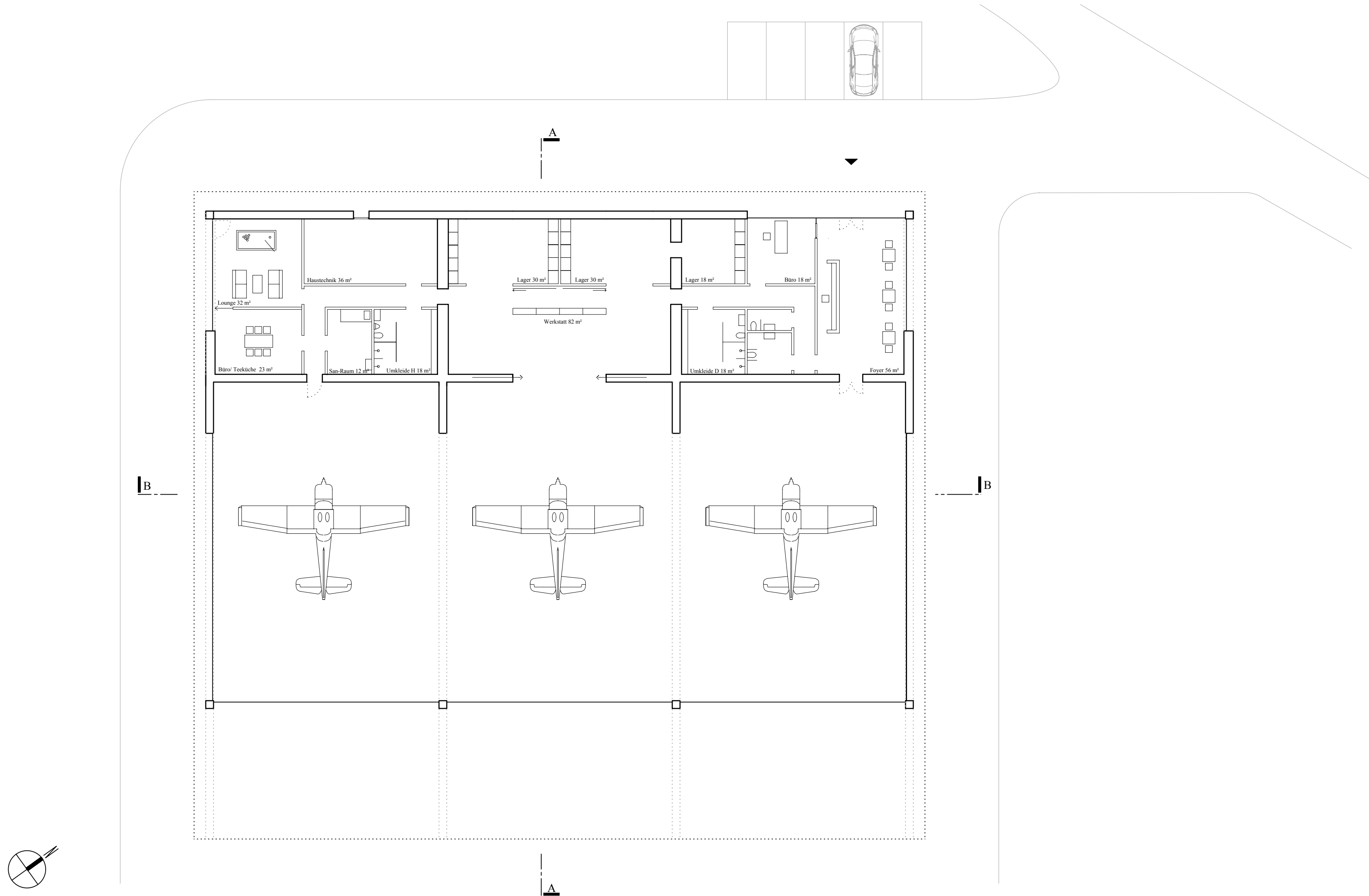
Grundriss M 1:200
