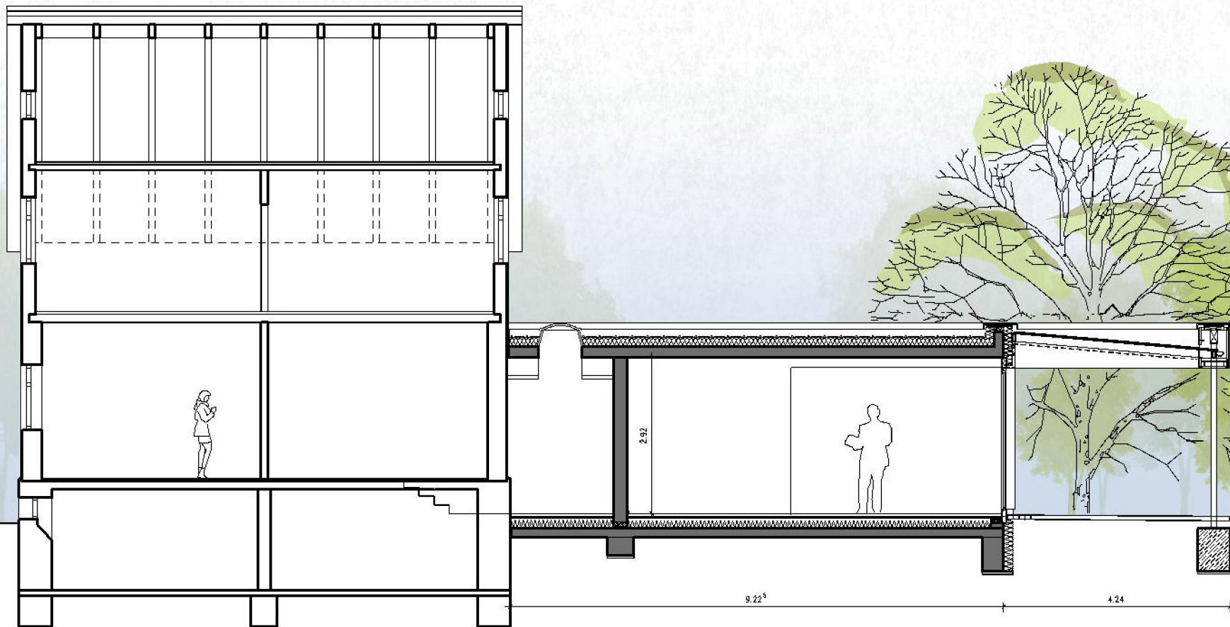
SCHNITT A - A
